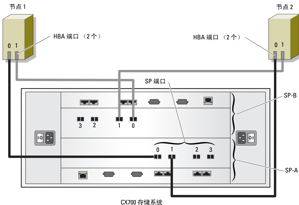
图 1-2. 直接连接光纤信道群集布线
